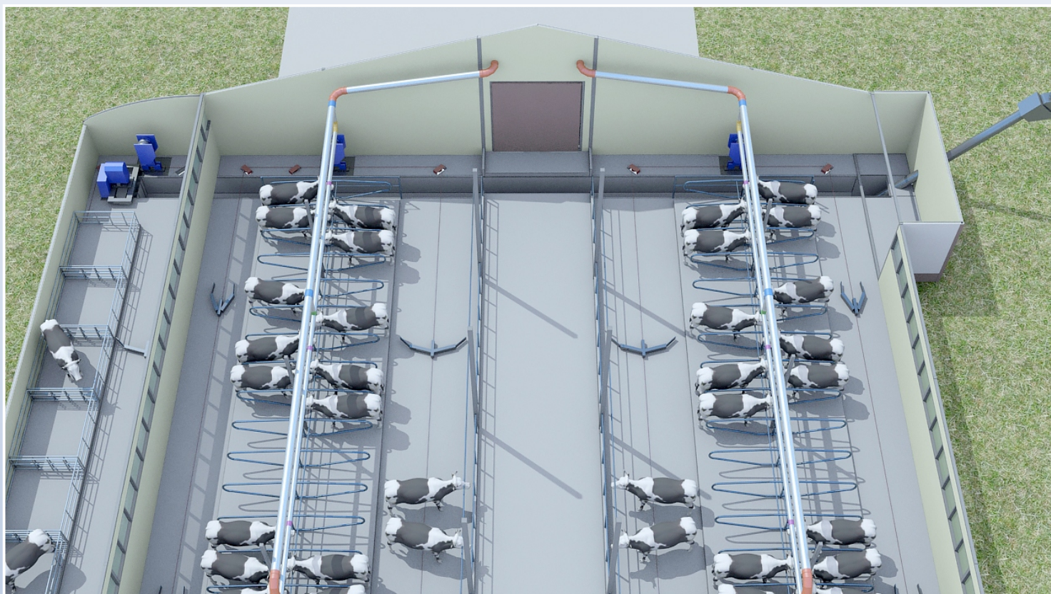
СИСТЕМА НАВОЗОУДАЛЕНИЯ
